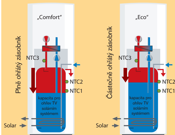
Schéma funkce Eco pro přípravu teplé vody
