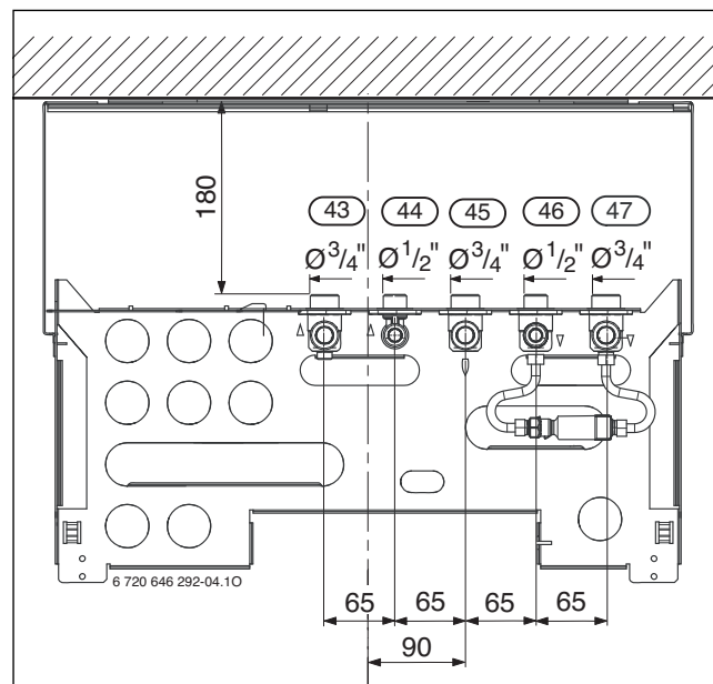
Obr. 11 Připojovací rozměry
